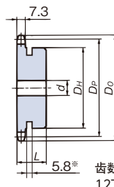
轮毅带凹槽(齿数12T)
