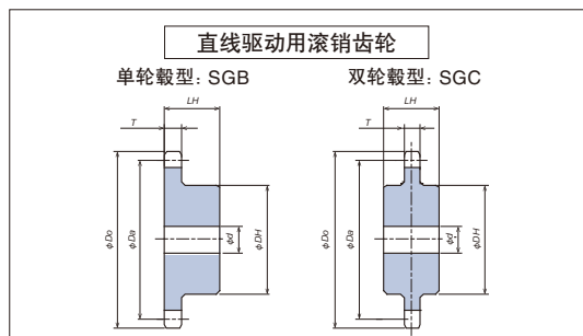
■ 销齿条・直线驱动用滚销齿轮尺寸表③ (PDU120~PDU240)
