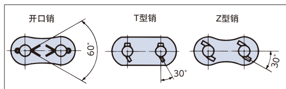
图11. 开口销等的开脚
