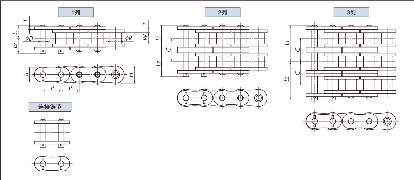
尺寸、规格
