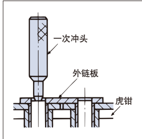
图4. 使用一次冲头锤击销子
