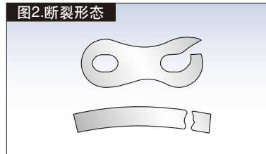
图2.断裂形态
