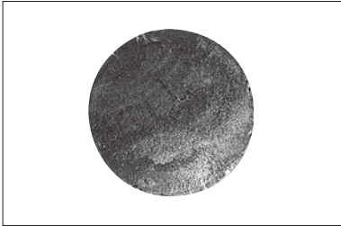
② 疲劳断裂 在反复承受超过销子的疲劳限度的大负荷 后，销子发生疲劳破坏的情形。再次检查高 峰负荷的大小并制定对策。
