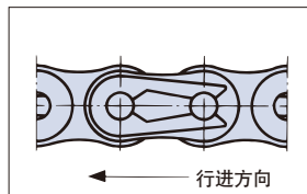
图10. 卡簧的安装方向
