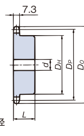
轮毅无凹槽(齿数13T以上)
