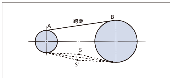
图15. 松弛量
