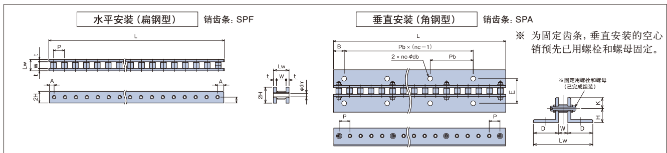
■ 销齿条·直线驱动用滚销齿轮尺寸表② (PDU050~PDU090)
