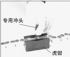
图7. 塑料组合链条的分解
