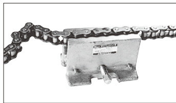
图3. 在链条虎钳上安装滚子链
