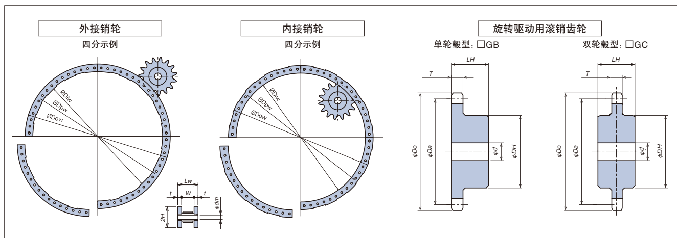
■ 销轮・旋转驱动用滚销齿轮尺寸表③ (PDU120~PDU240)
