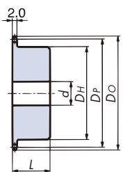
(切削加工规格) 1B型
