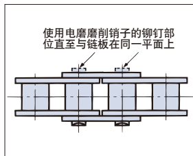
图1. 铆接形式滚子链
