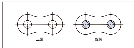
图27. 销子的旋转
