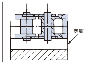
图6. 将塑料组合链条安装在虎钳上
