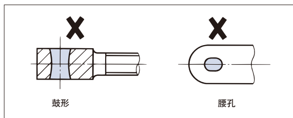
图33. 末端固定工具的孔的磨损
