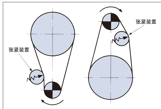
图23. 垂直传动时的调整例
