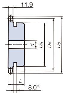
轮毂带凹槽 (齿数10T~11T)
