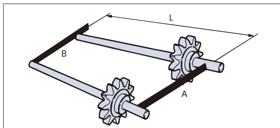
图17. 轴的平行度
