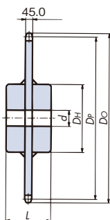
(焊接规格) 1C型
