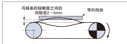
图22. 防振导向挡块
