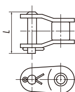
1节距型过渡链节
