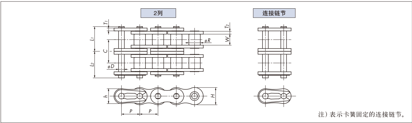
尺寸、规格
