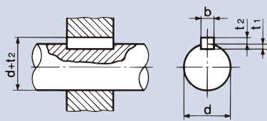
平行键 (JIS B 1301-1959)
