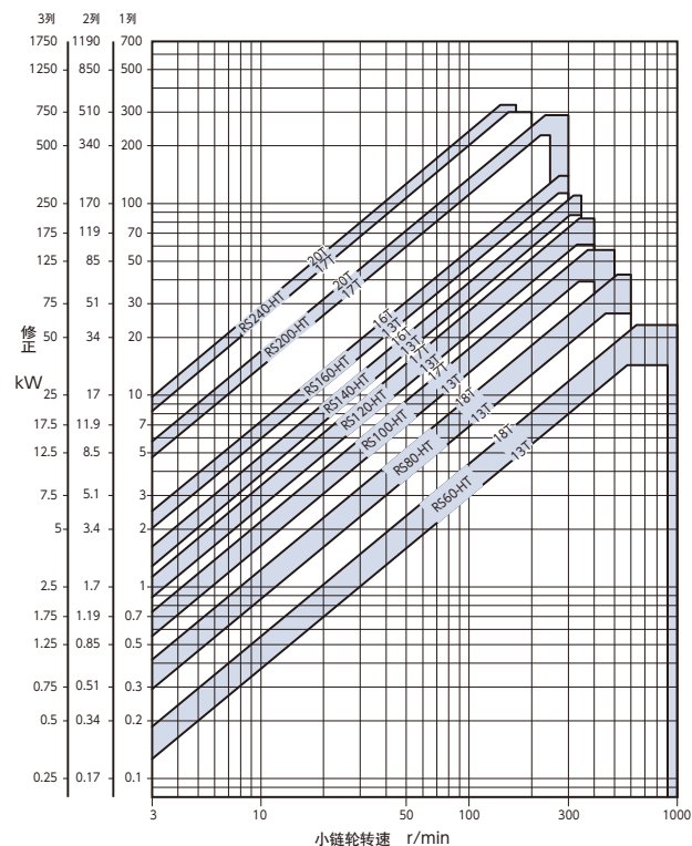
图3 高强度链条RS-HT简易选型图
