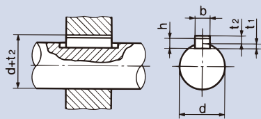
平行键 (JIS B 1302-1996)
