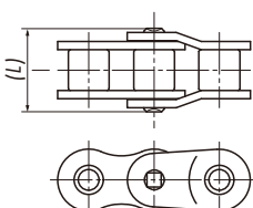
2节距型过渡链节
