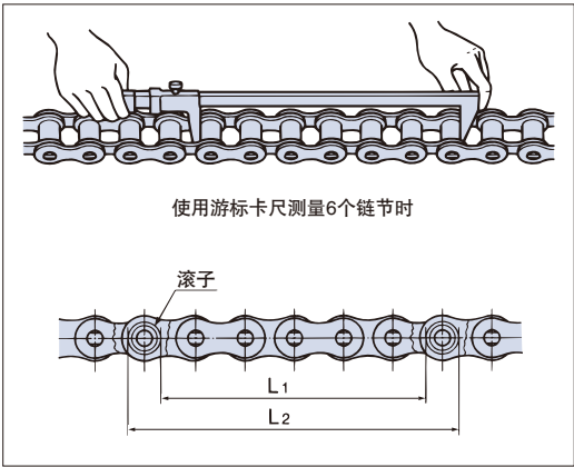
图31. 长度的测量
