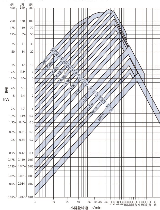
图5 RS滚子链条BS/DIN规格简易选型图
