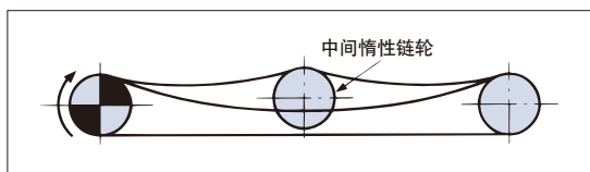
图21. 中心距离长时的调整例
