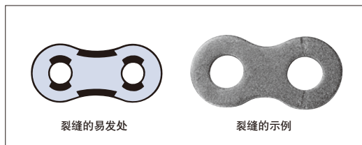
图25. 链板的裂缝
