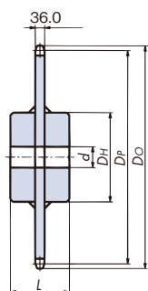
(焊接规格) 1C型
