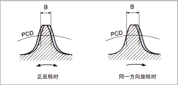
图30. B尺寸的位置
