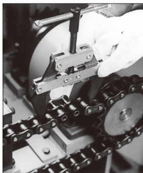
图9. 在轴间连接
