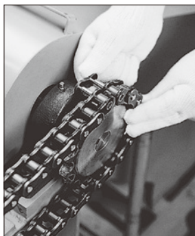
图8. 在链轮部连接
