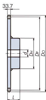
(焊接规格) 1B型
