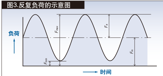
图3.反复负荷的示意图
