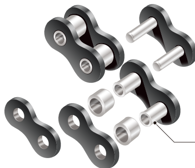
LAMBDA链 基本构造
