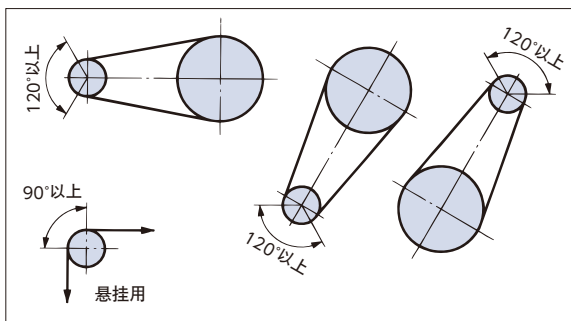
图13. 缠绕角度
