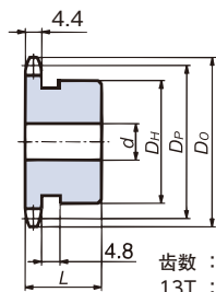
轮毅带凹槽(齿数13T)
