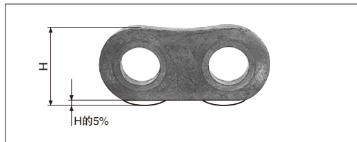
图26. 链板端面的磨损
