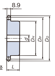
轮毅无凹槽(齿数14T以上)
