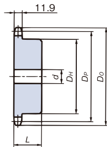
轮毂无凹槽 (齿数12T~30T)
