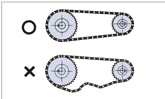
图14. 松弛例
