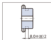
吊孔尺寸
