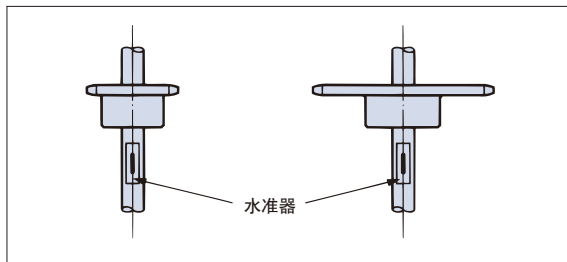
图16. 轴的水平度
