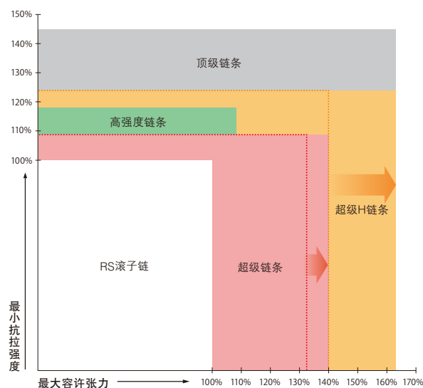
最小抗拉强度・最大容许张力的比较
