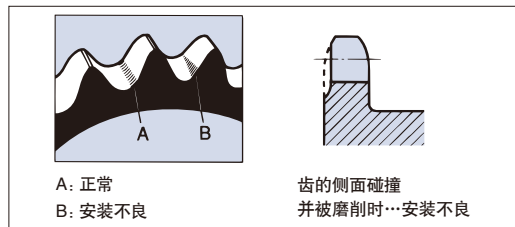
图29. 链轮齿面的碰撞
