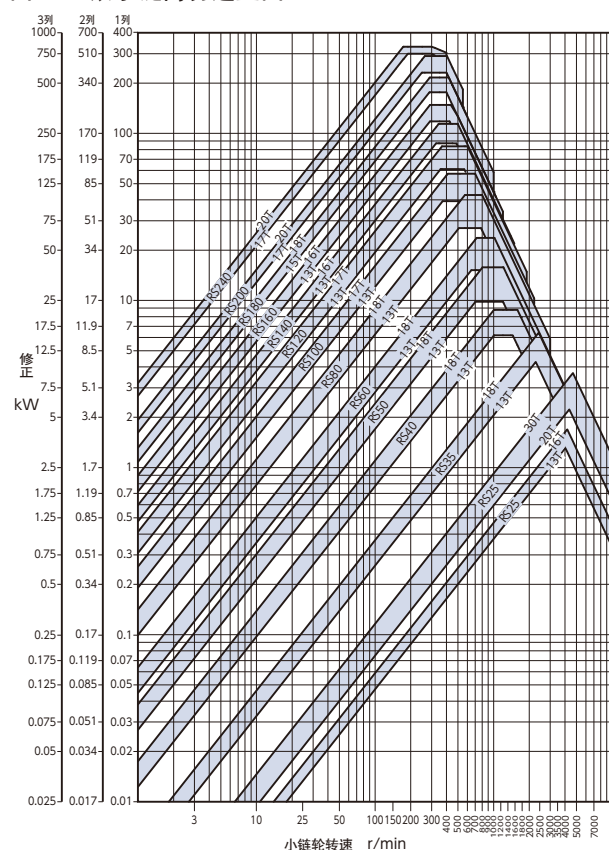
图3 高强度链条RS-HT简易选型图
