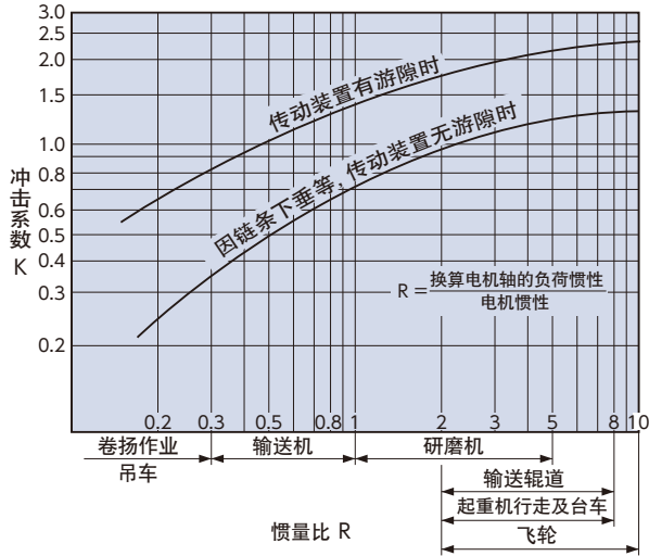
图1 冲击系数 K
