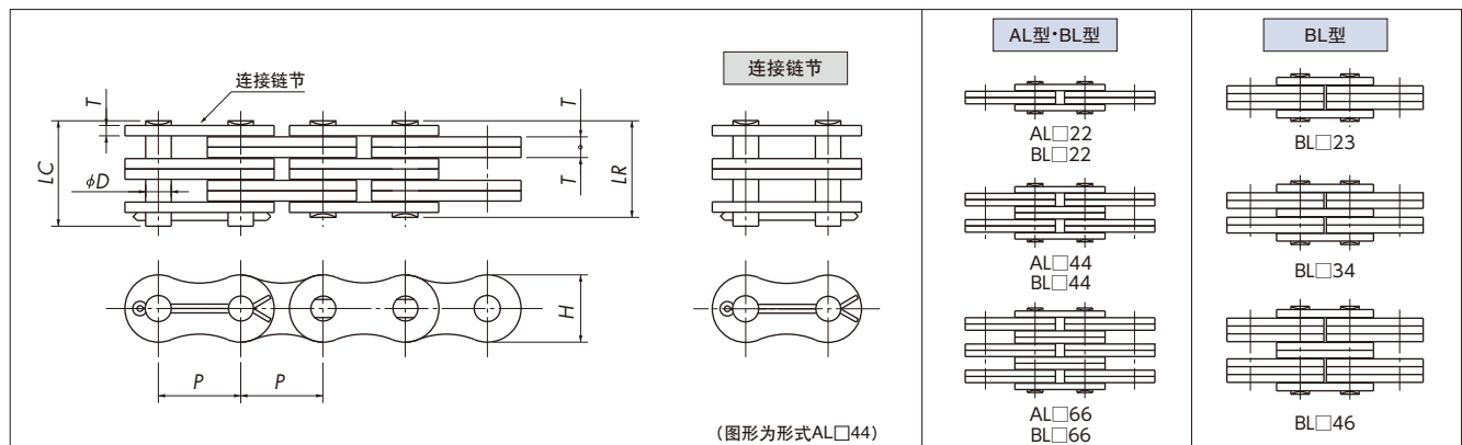
■ AL型的尺寸、规格
