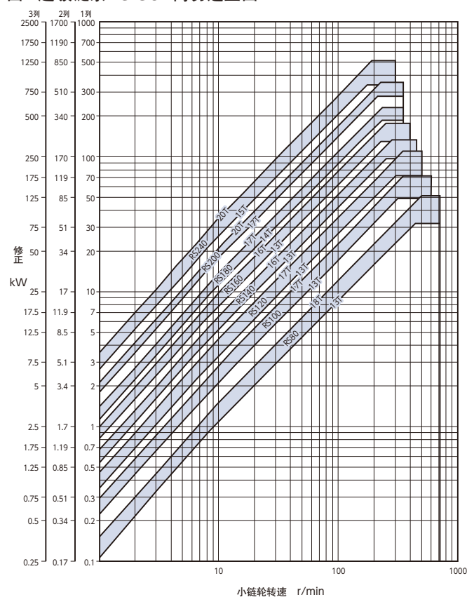
图1 超级链条RS-SUP简易选型图
