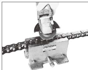
图2. 打磨销子的端部
