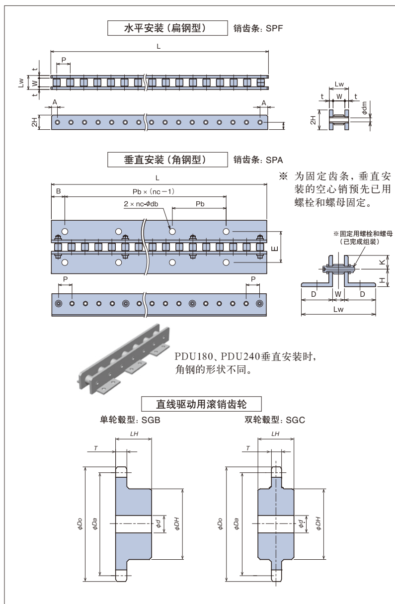
滚销齿轮
