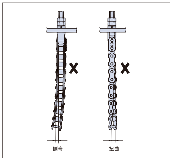
图32. 滚子链的扭曲
