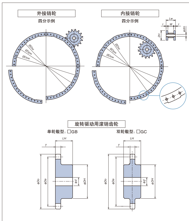
滚销齿轮
