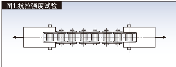
图1.抗拉强度试验
