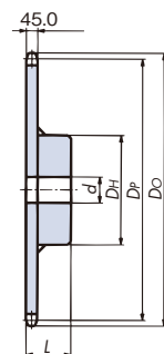
(焊接规格) 1B型
